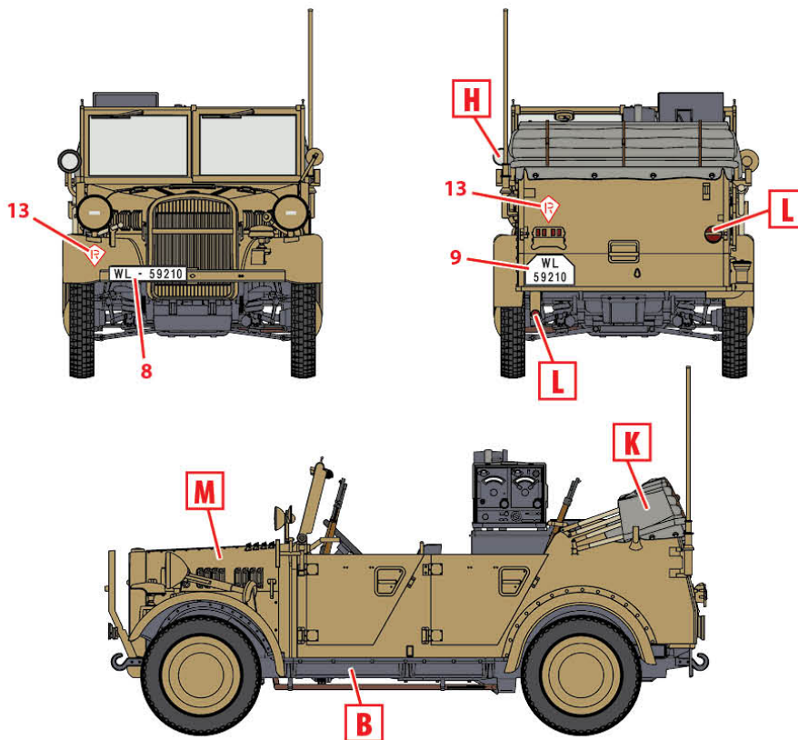
4. le.gl.Einheits-Pkw (Kfz.2), бригада Рамке, Лівія, 1942 р. le.gl.Einheits-Pkw (Kfz.2), Ramcke Brigade, Libya, 1942
