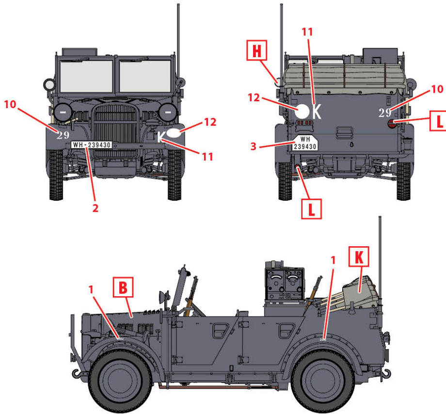
1. le.gl.Einheits-Pkw (Kfz.2), 29-й артполк, Франція, червень 1940 р. le.gl.Einheits-Pkw (Kfz.2), 29th Artillery Regiment, France, June 1940
