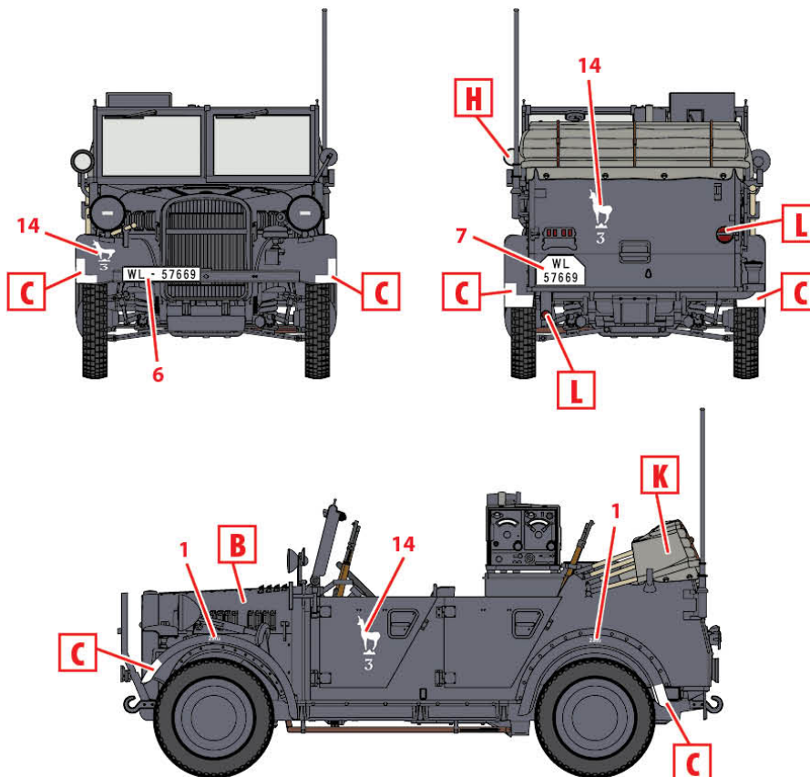
2. le.gl.Einheits-Pkw (Kfz.2), 3./JG 51, Смоленськ (Росія), август 1941 г. le.gl.Einheits-Pkw (Kfz.2), 3./JG 51, Smolensk (Russia), August 1941
