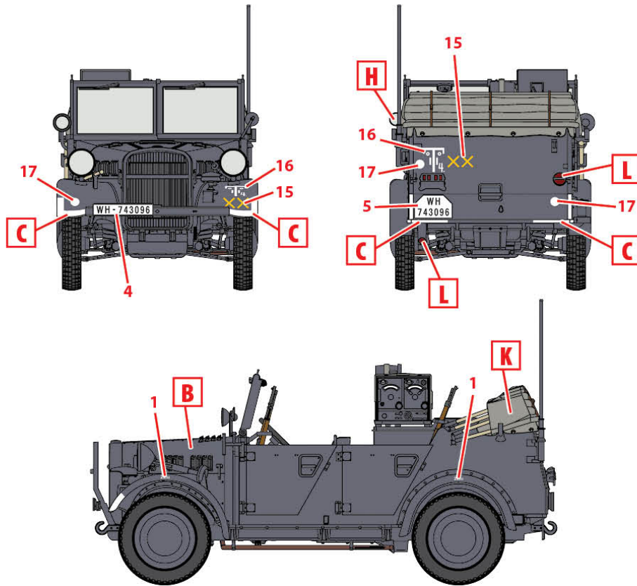
3. le.gl.Einheits-Pkw (Kfz.2), 6-та танкова дивізія, Росія, вересень 1941 р. le.gl.Einheits-Pkw (Kfz.2), 6 P.D., Russia, September 1941
